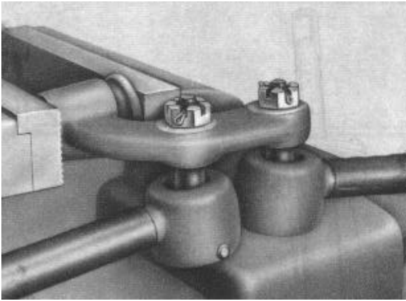
Bild F 6. Spurstangen abbauen
