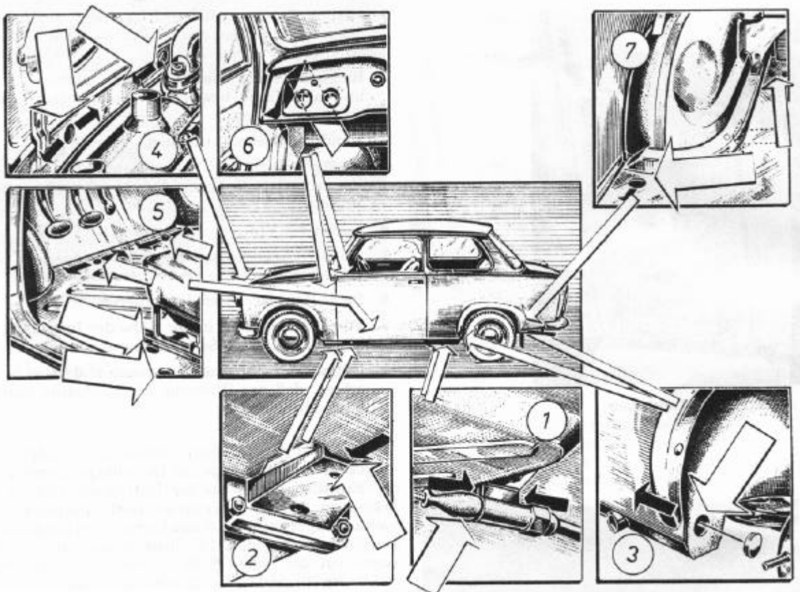
Bild K 24. Hohlraumkonservierung Hohlraum
