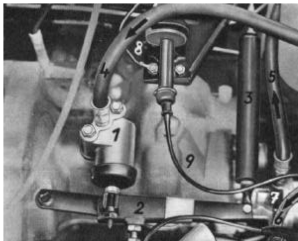
Bild H 16. Aggregate am Getriebe (1) Kupplungszyylinder (2) Kupplungshebel (3) Rückzugfeder (4) Druckschlauch vom Steuerventil (6) Druckschlauch zum Steuerventil (6) Schlauch vom Vorratsbehälter (7) Hydraulikpumpe (8) Masseleitung (9) Kabel vom Schalthebel zum Relais
